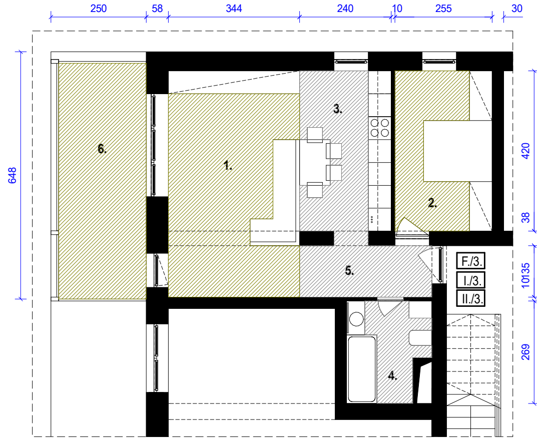
ALAPRAJZ M = 1:100
