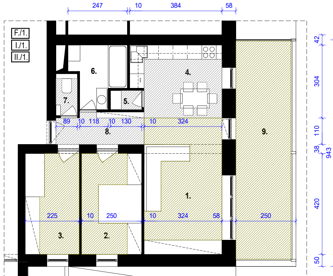
ALAPRAJZ M = 1:100
